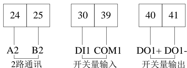
图 7 通讯、开关量接线
