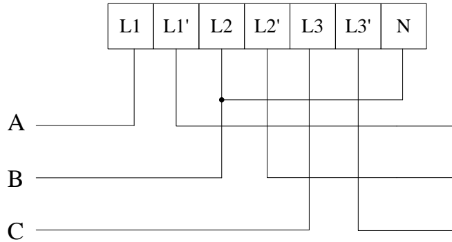
图 5 三相三线直接接入
