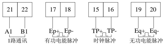
图 6 通讯、脉冲接线
