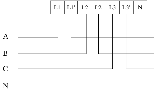
图 3 三相四线直接接入
