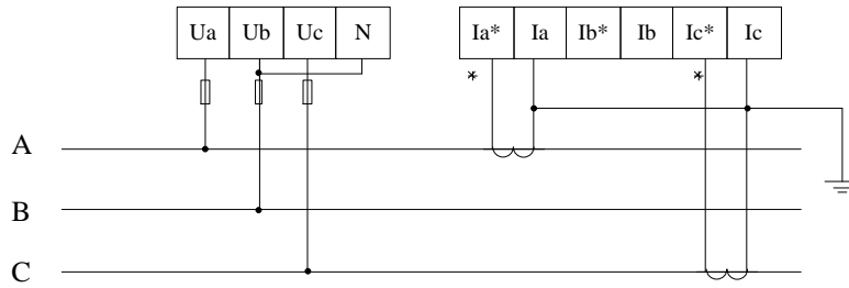
图 4 三相三线经互感器接入
