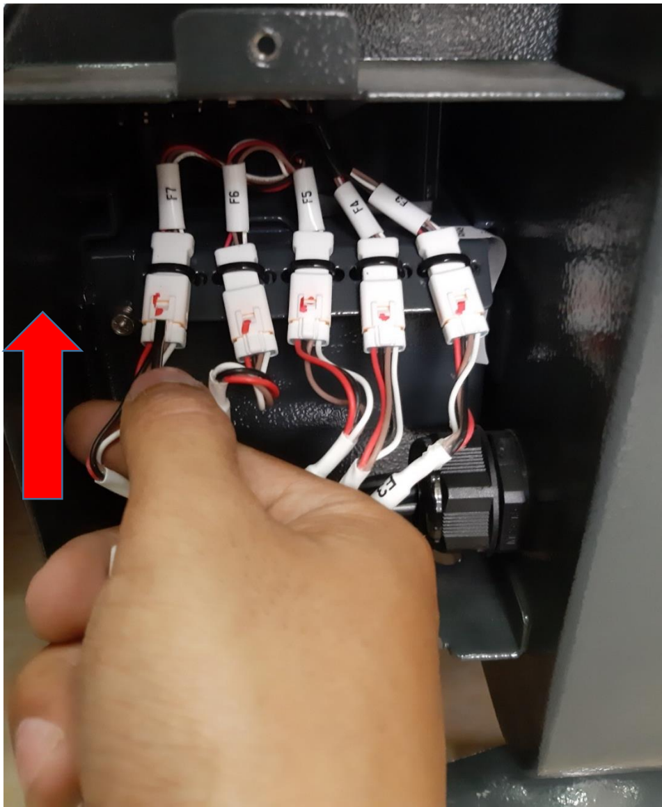
Lắp khay quạt vào inverter
